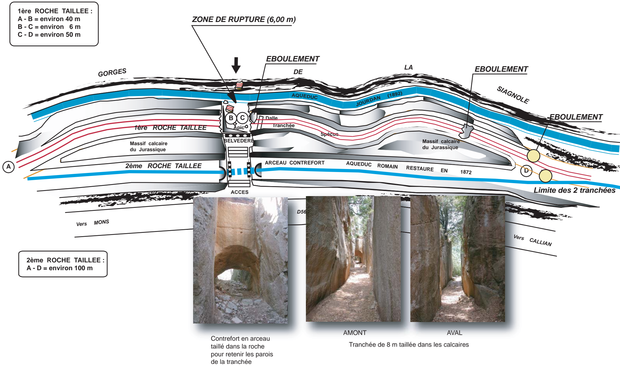
Ce schéma n'est pas à l'échelle, il s'étend sur une longueur de 100 m environ
